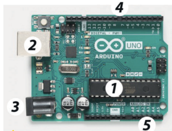
1 Carte Arduino dont les éléments importants sont identifiés
