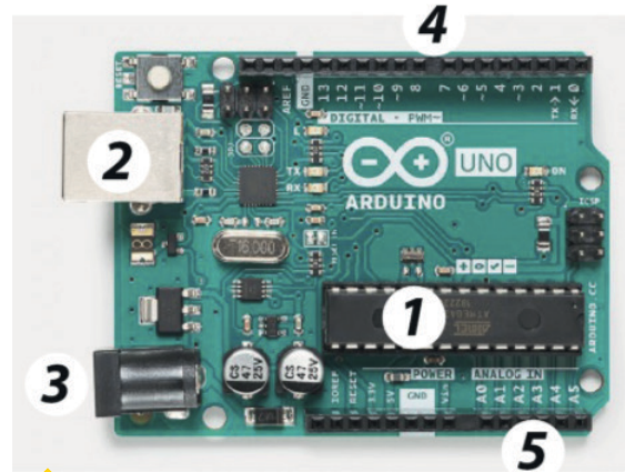
1 Carte Arduino dont les éléments importants sont identifiés
