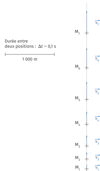
Situation n° 1. Positions successives de la fusée.
