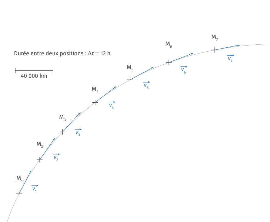
Situation n° 2. Positions successives de la Lune.
